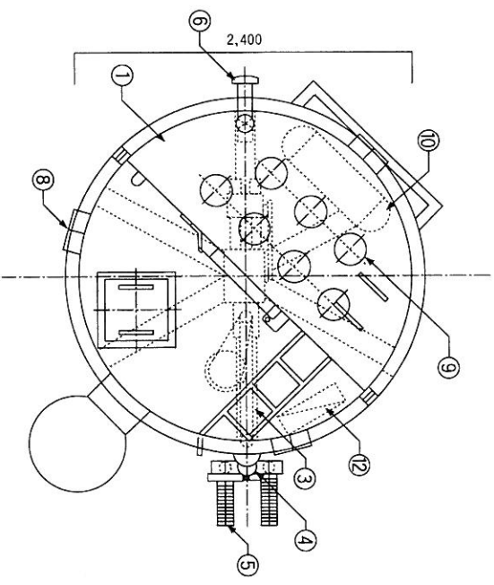
セメントサイロ平面図 S1/20
